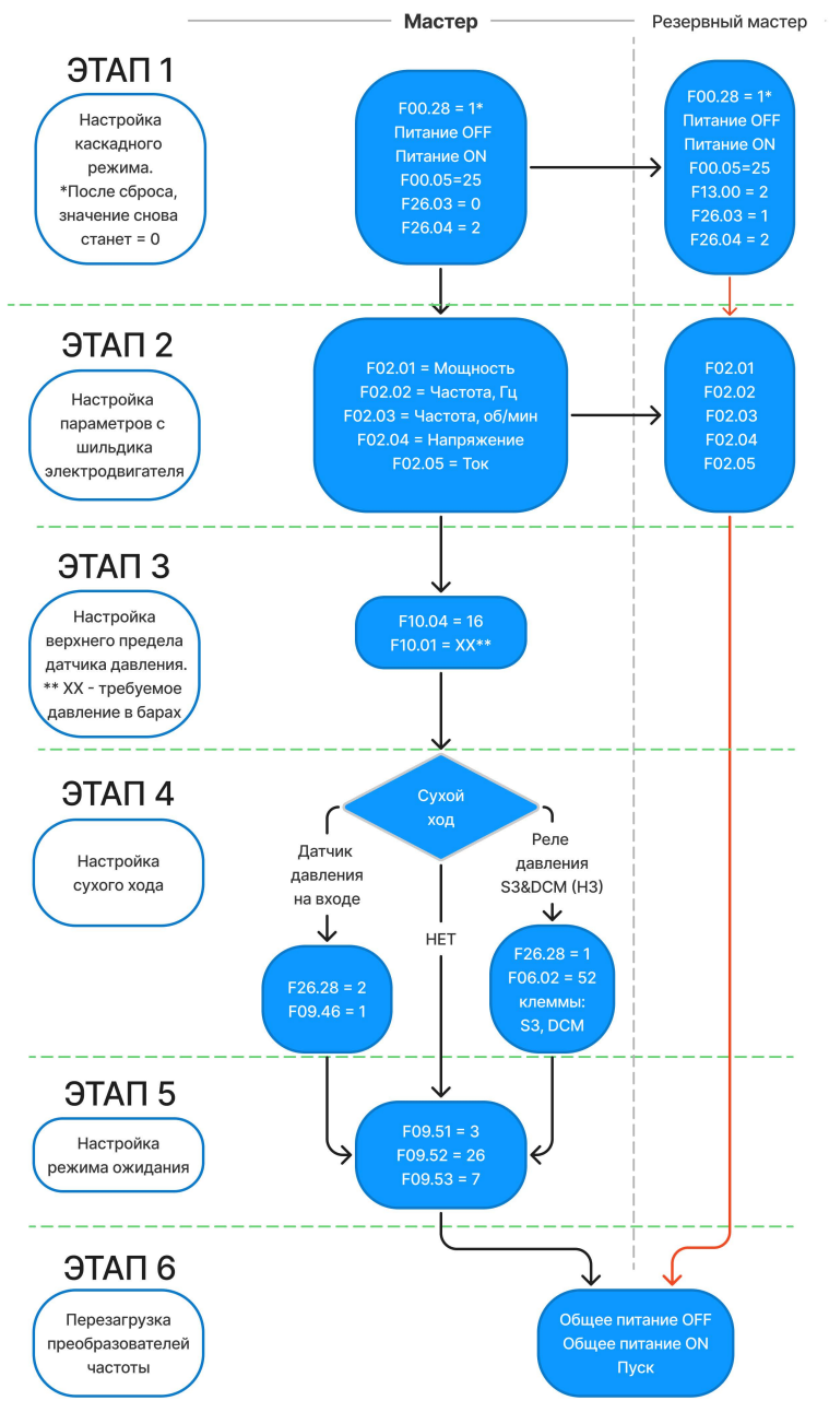
Рис. 12 Пример настройки 2-х насосной станции
