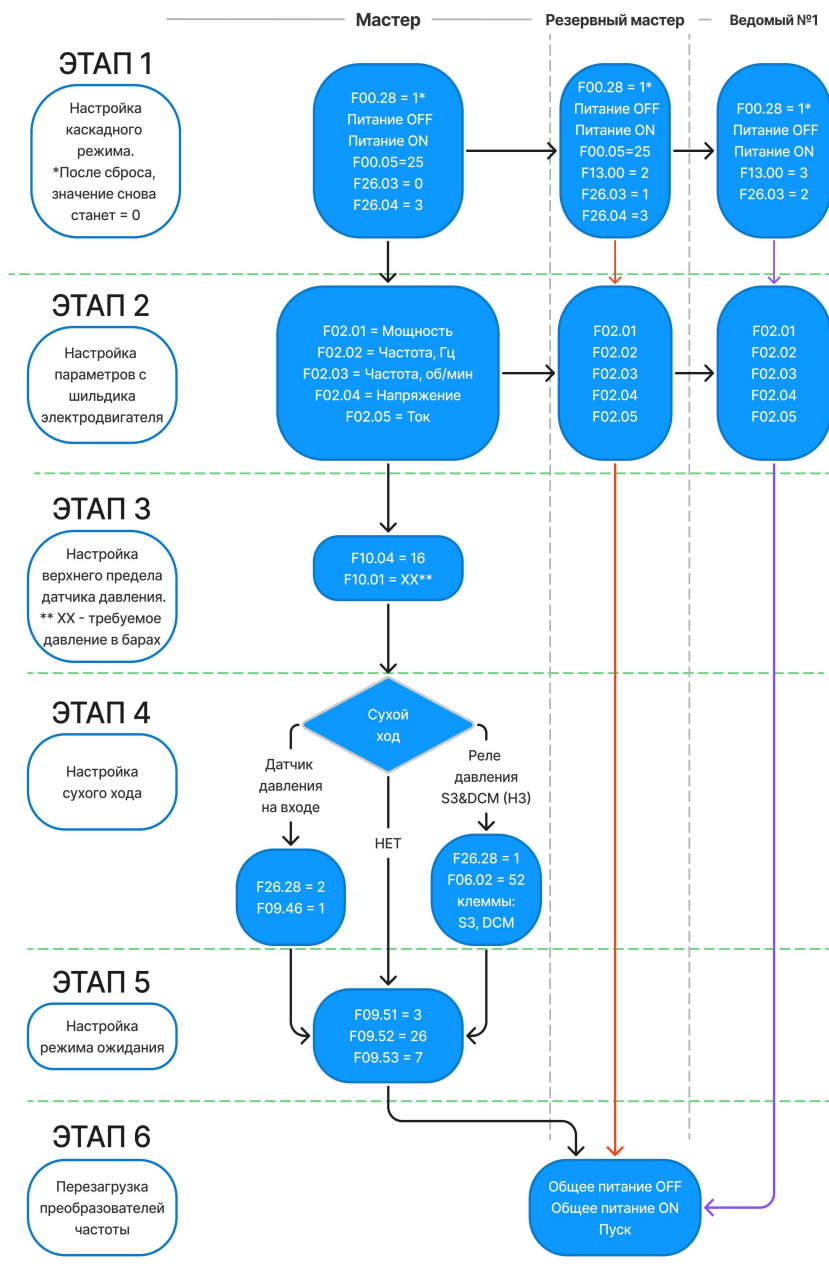
Рис. 13 Пример настройки 3-х насосной станции
