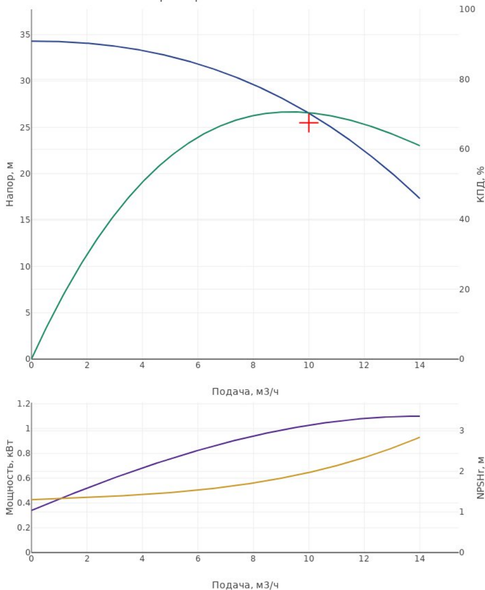
Характеристика насоса CDM10-3
