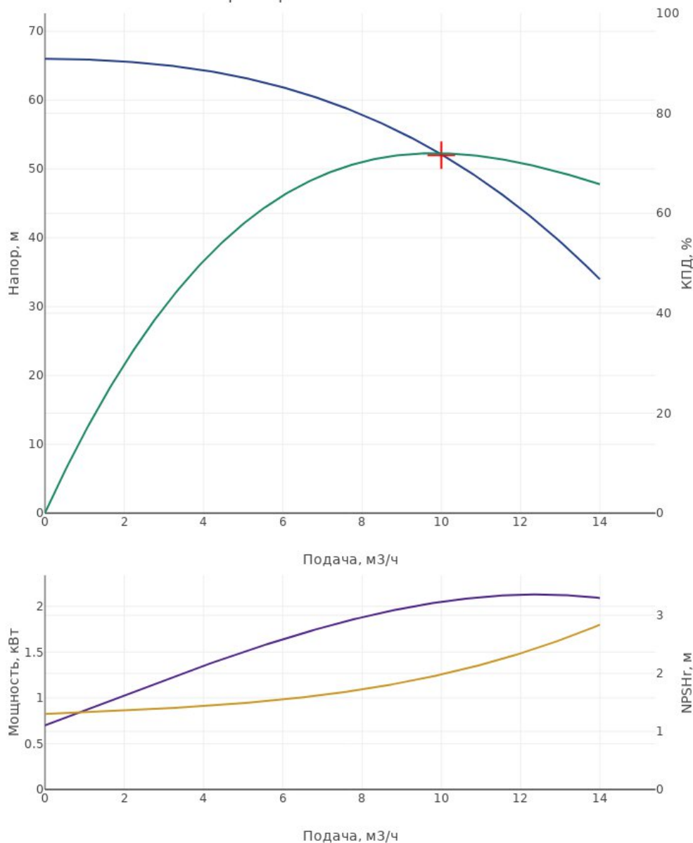
Характеристика насоса CDM10-6
