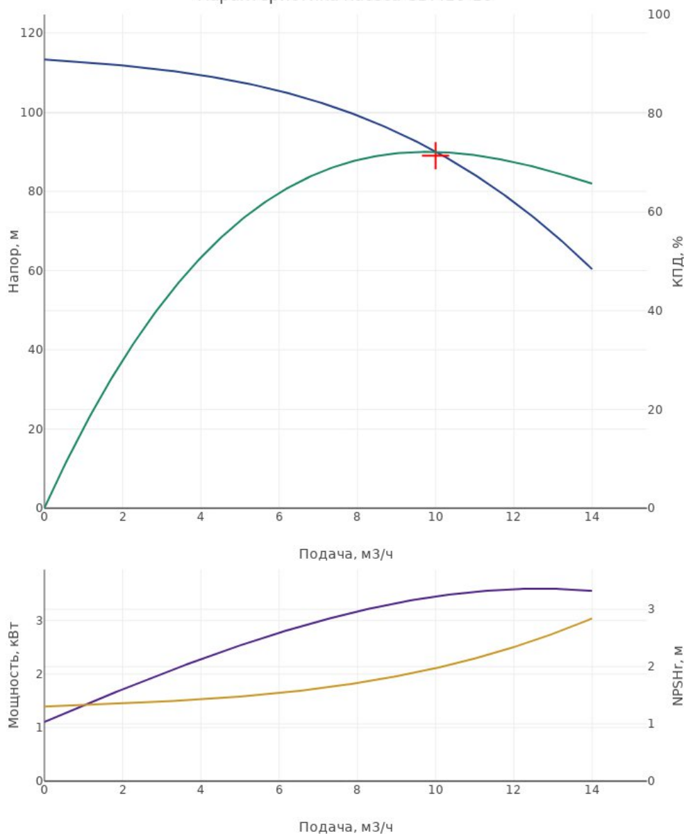
Характеристика насоса CDM10-10
