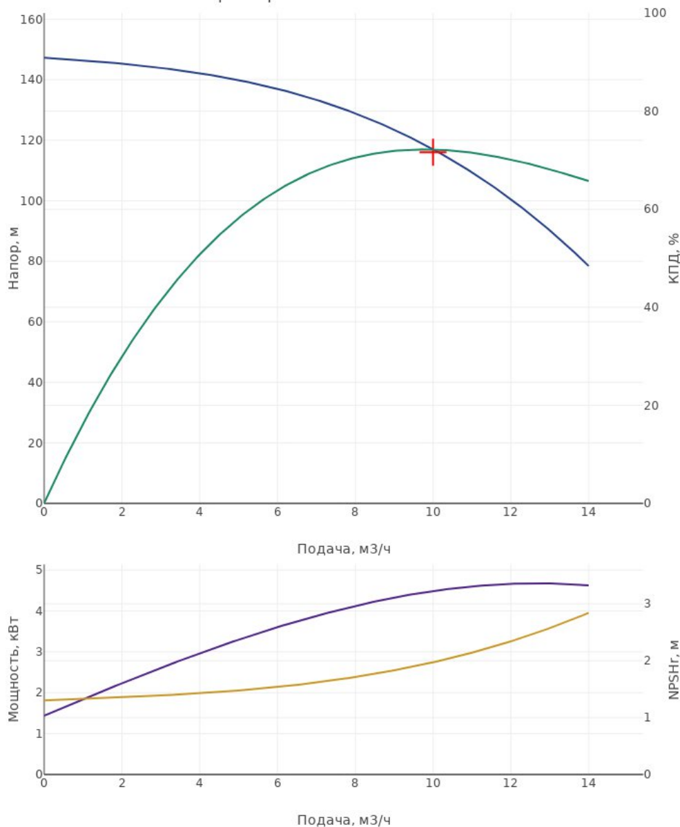
Характеристика насоса CDM10-13
