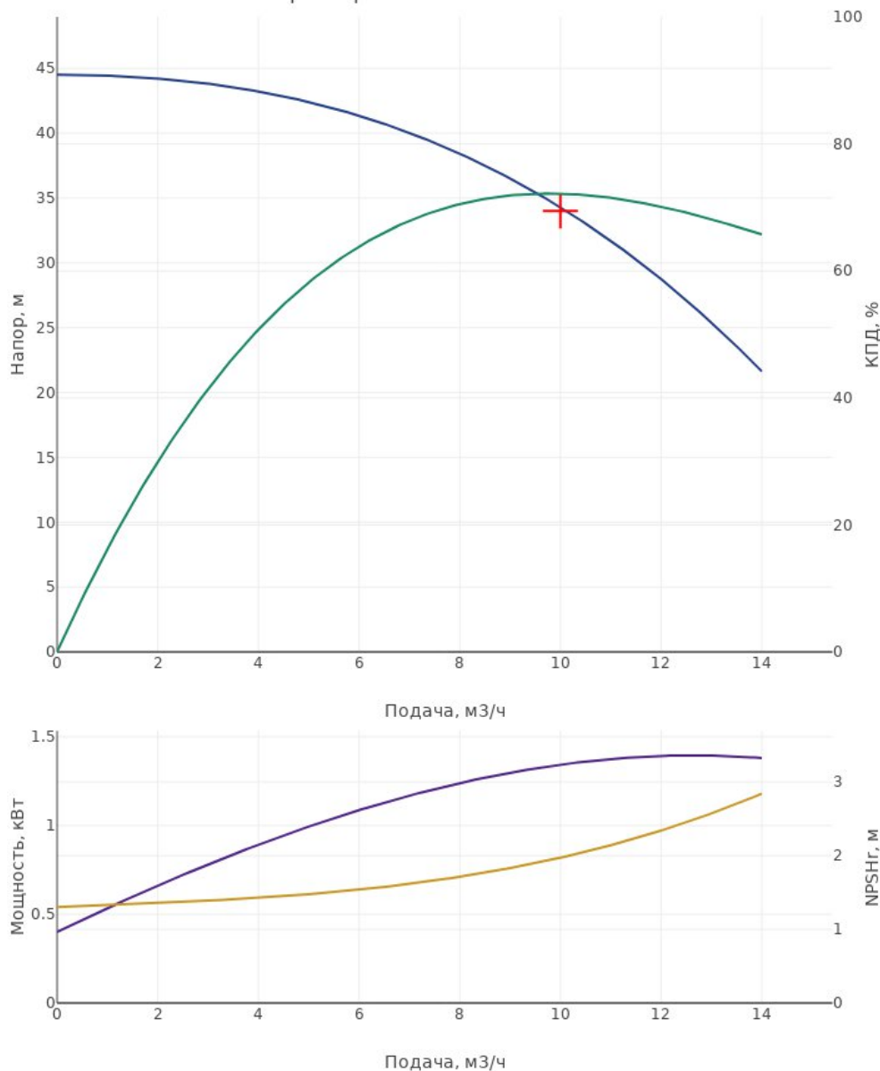
Характеристика насоса CDM10-4
