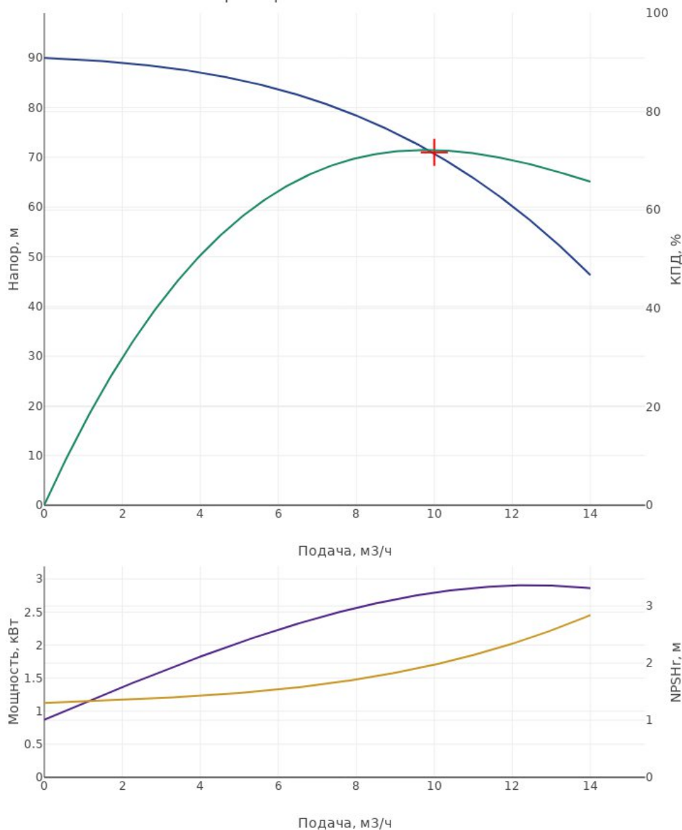
Характеристика насоса CDM10-8
