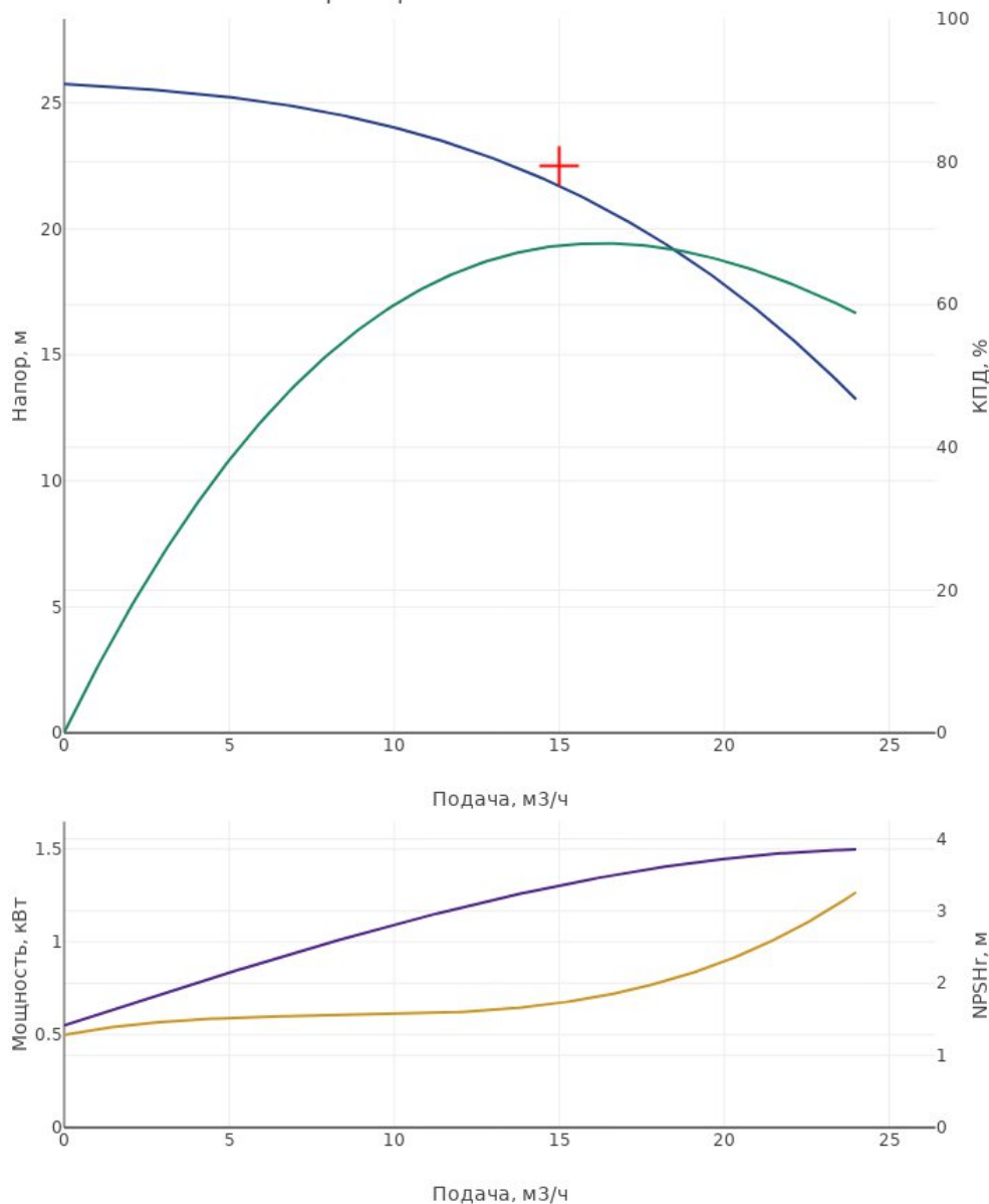
Характеристика насоса CDM15-2
