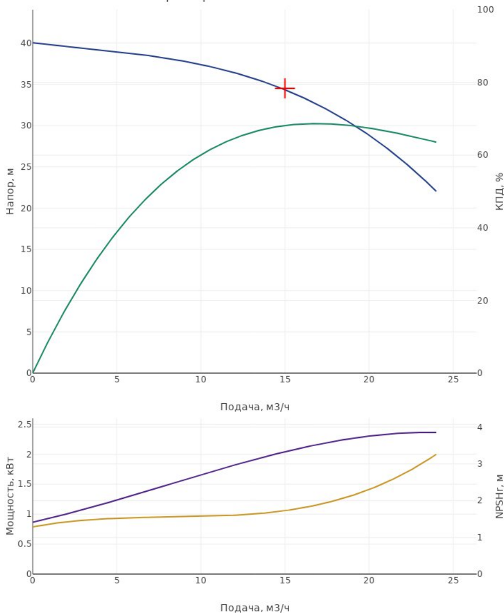
Характеристика насоса CDM15-3
