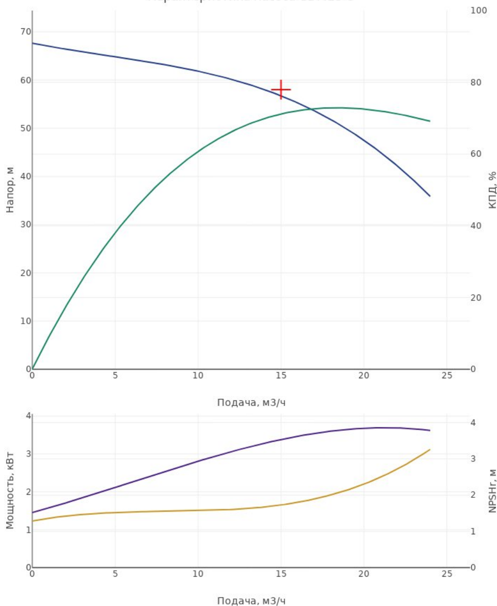
Характеристика насоса CDM15-5
