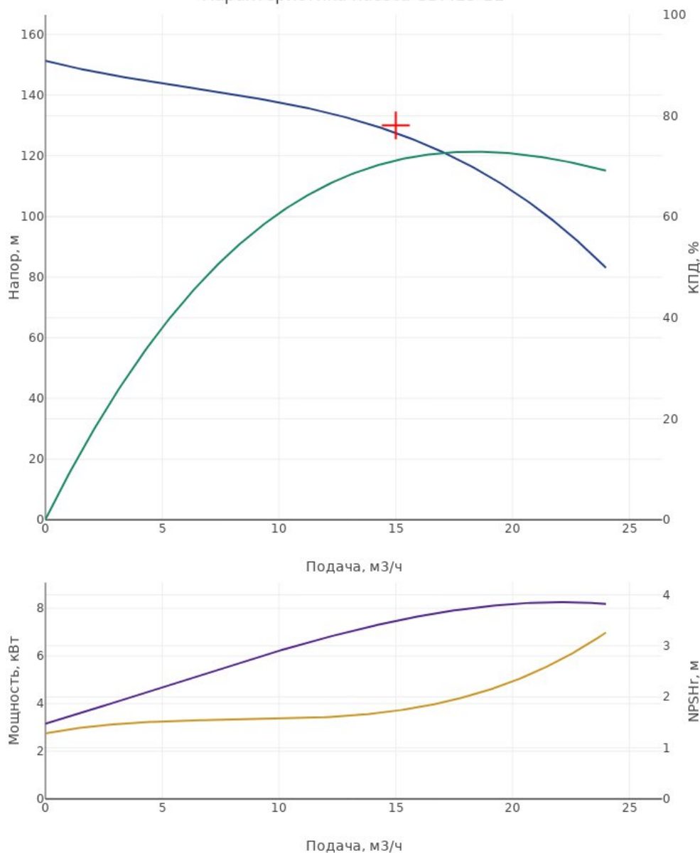
Характеристика насоса CDM15-11
