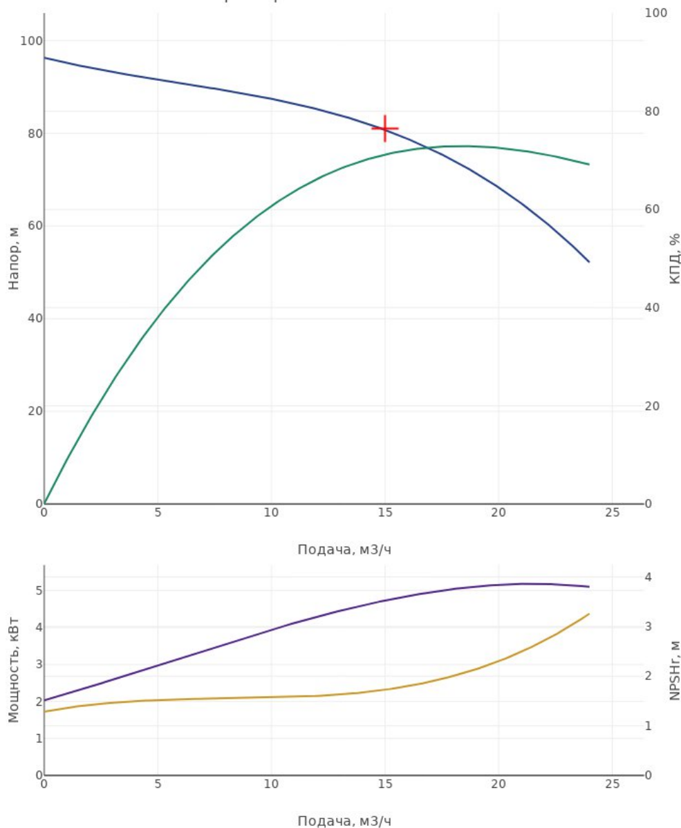
Характеристика насоса CDM15-7
