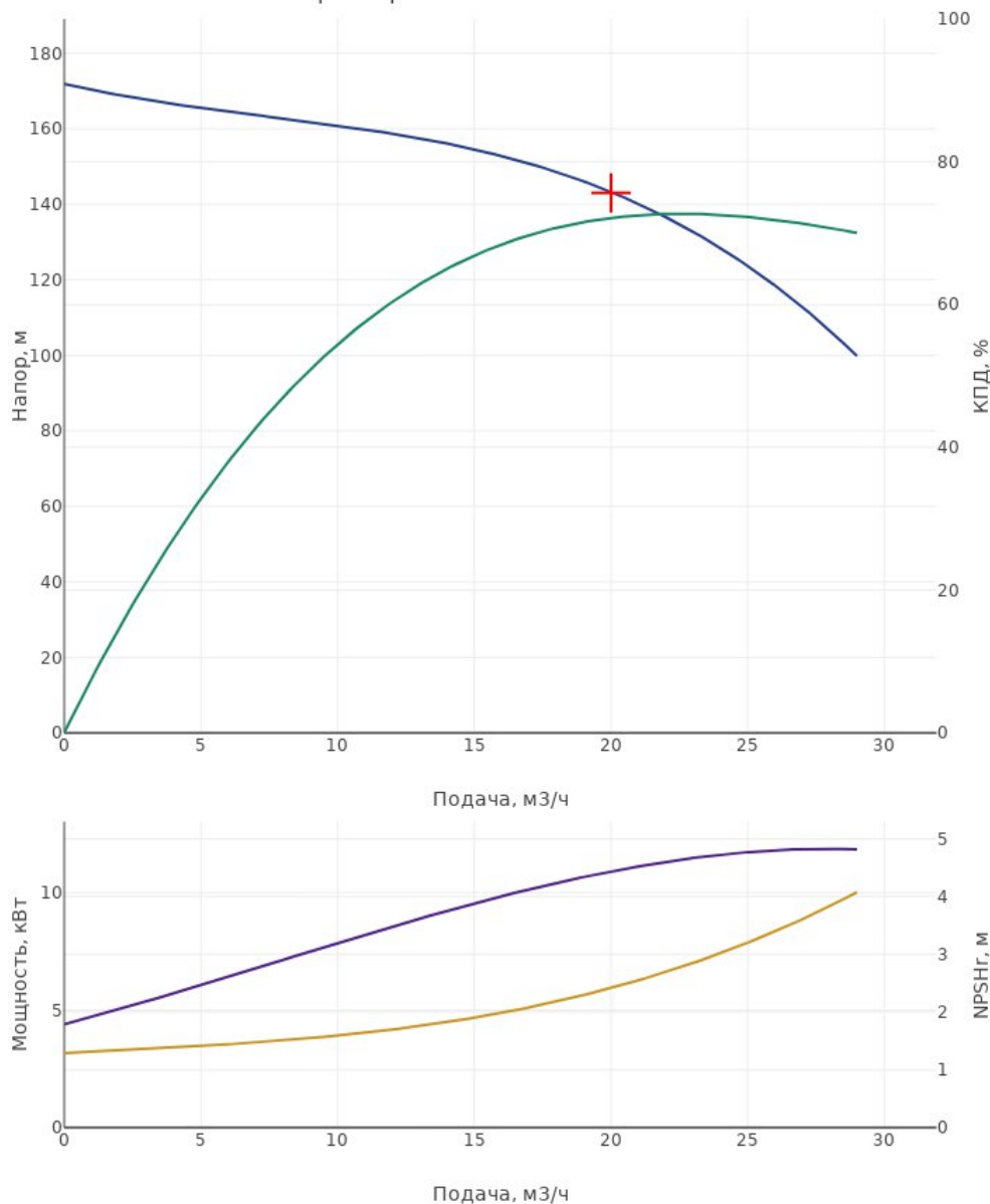
Характеристика насоса CDM20-12
