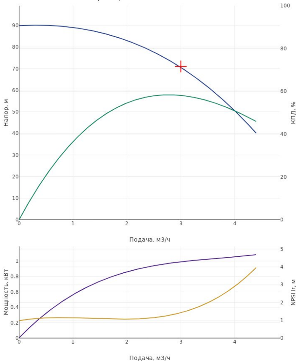
Характеристика насоса CDM3-12
