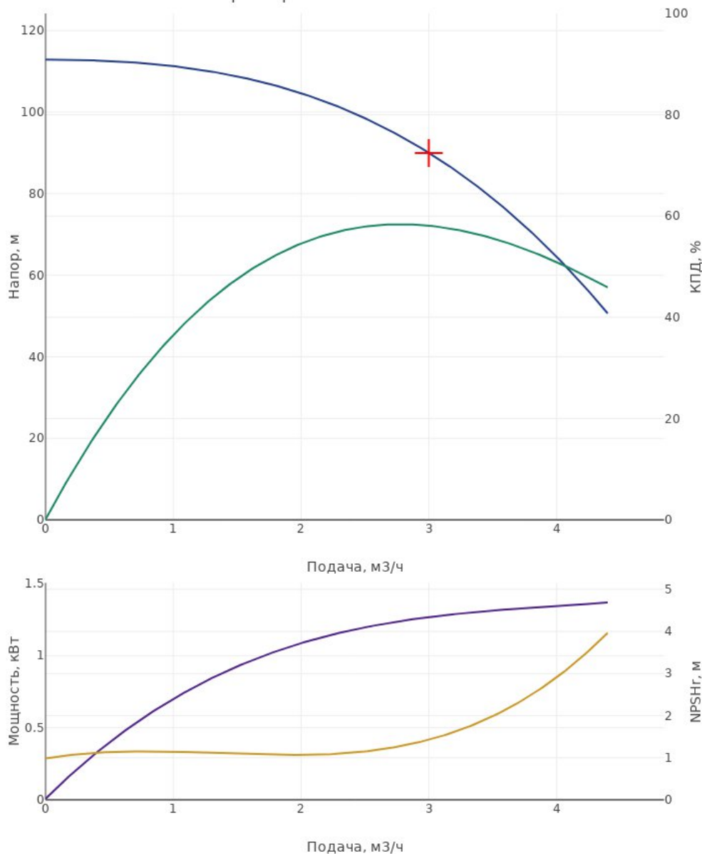
Характеристика насоса CDM3-15
