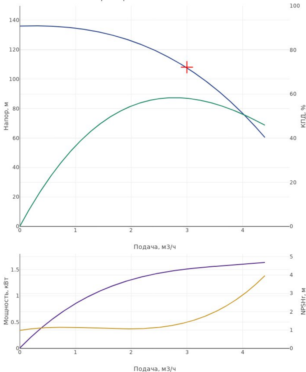
Характеристика насоса CDM3-18
