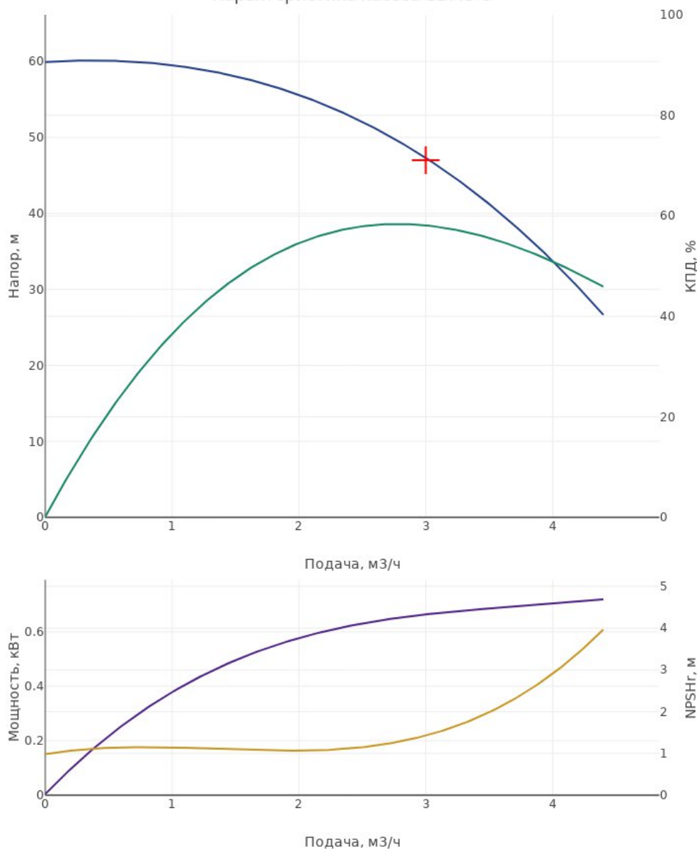
Характеристика насоса CDM3-8
