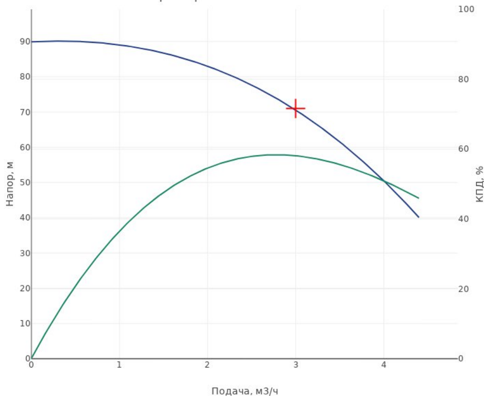
Характеристика насоса CDM3-12
