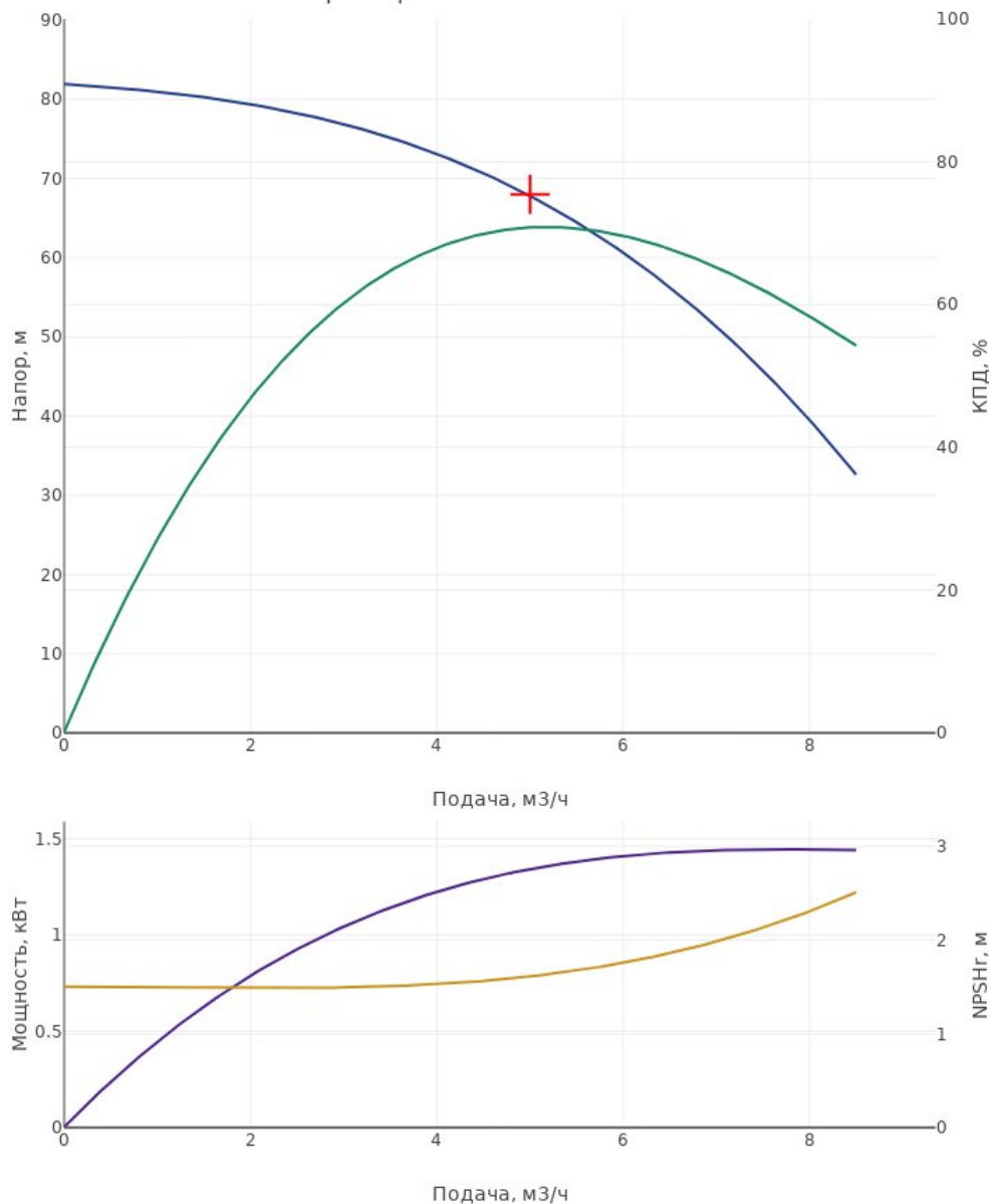
Характеристика насоса CDM5-11
