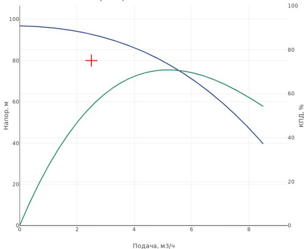
Характеристика насоса CDM5-13
