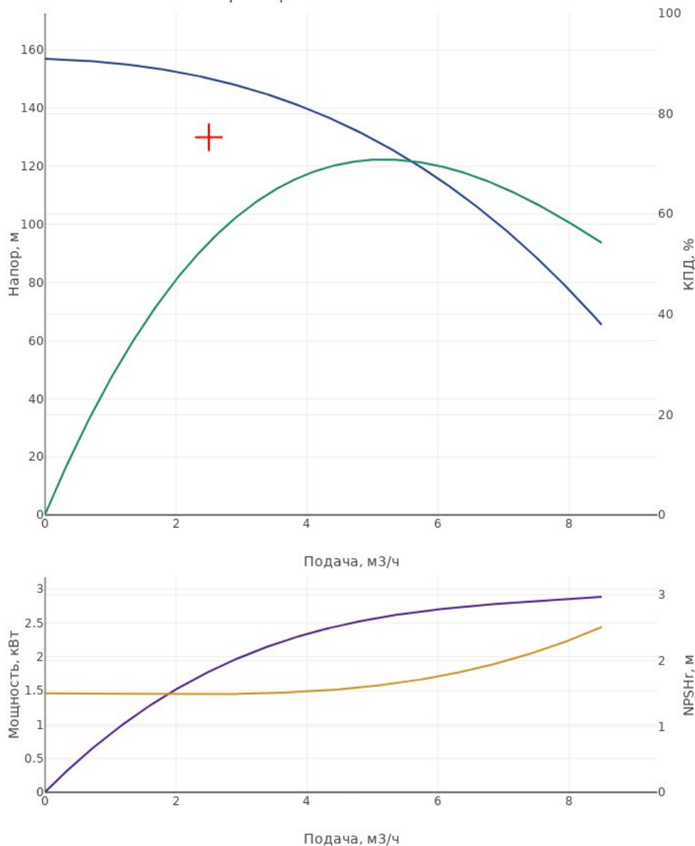
Характеристика насоса CDM5-21
