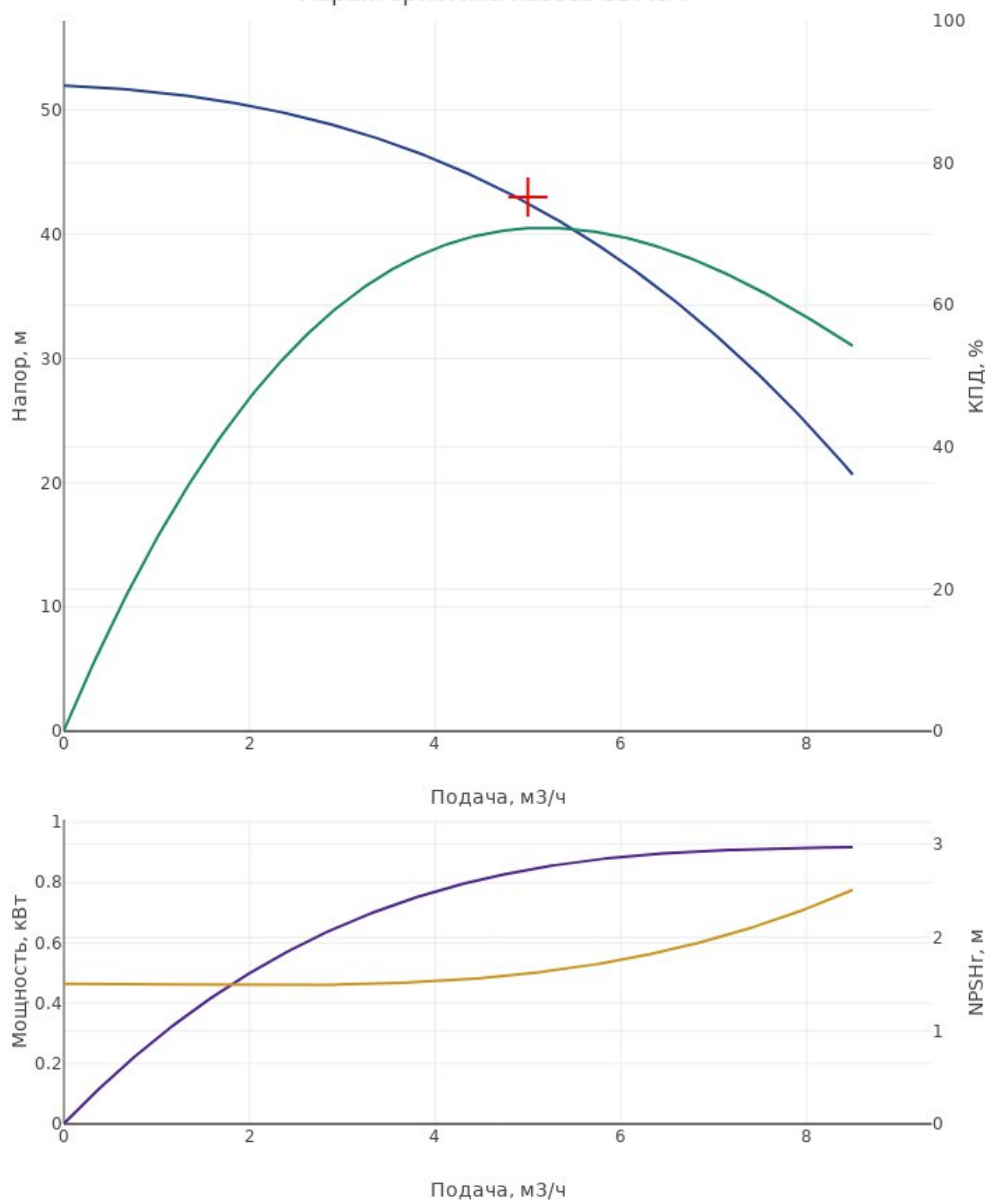
Характеристика насоса CDM5-7
