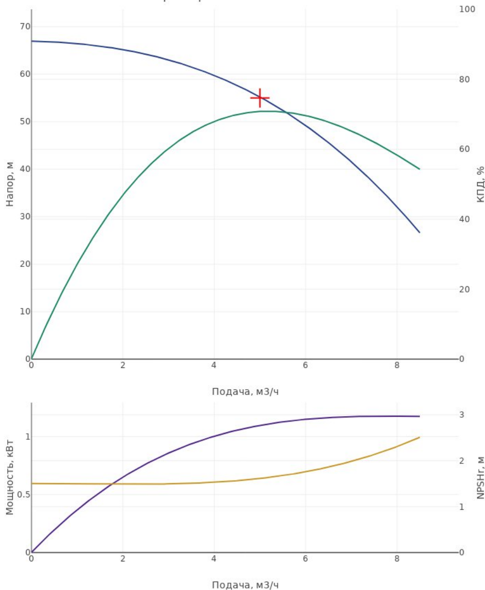
Характеристика насоса CDM5-9
