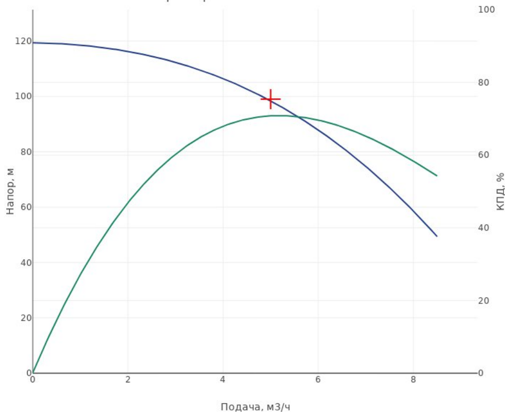
Характеристика насоса CDM5-16
