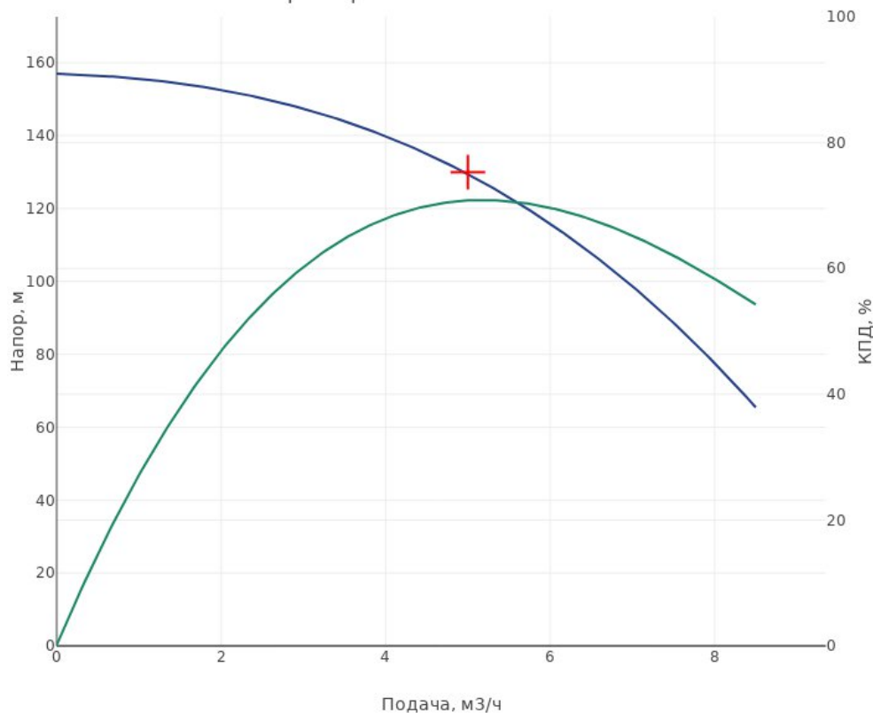
Характеристика насоса CDM5-21
