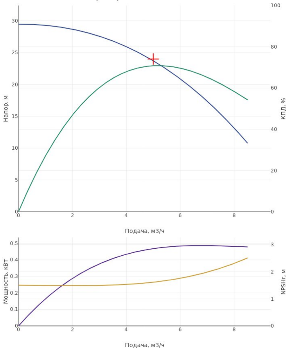
Характеристика насоса CDM5-4
