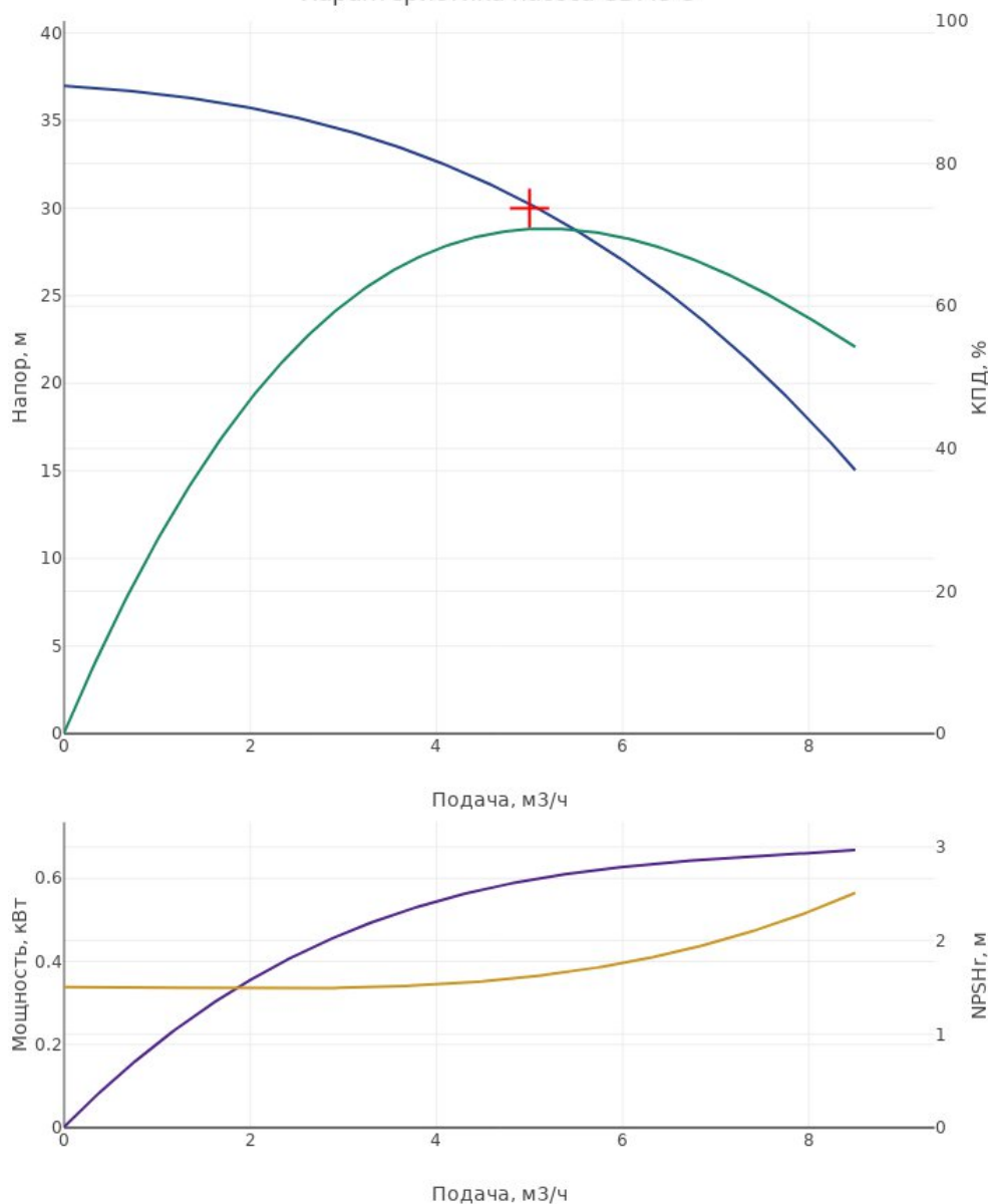
Характеристика насоса CDM5-5
