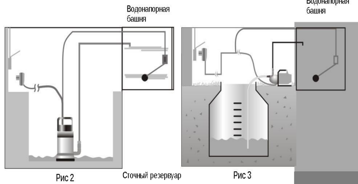
Водонапорная башня
